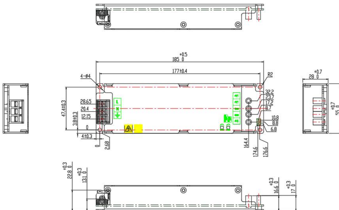
外形尺寸及安装孔——端子坐标图
